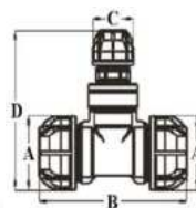
DESENHO TÉCNICO
